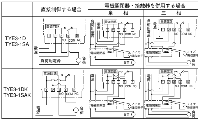
端子配置図
