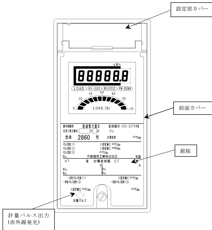
「普通電力量計正面図」
