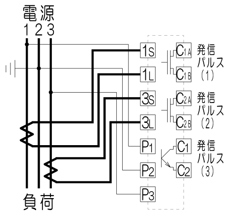
「単相 3 線式・三相 3 線式」 CT付
