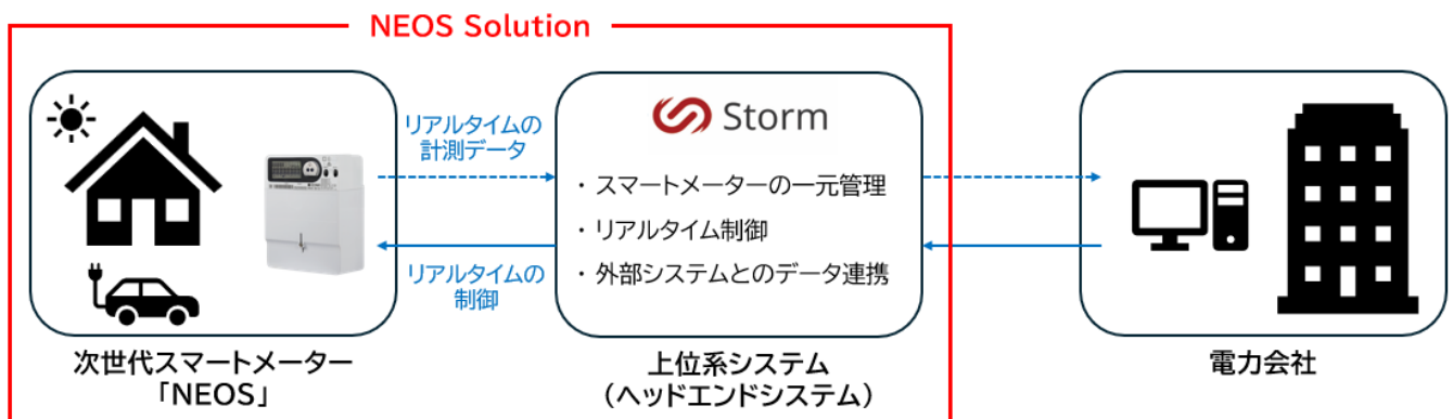
図1 <EDMI の「NEOS Solution」(ネオス ソリューション)のシステム概念図>
