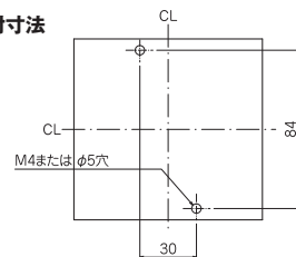
取付寸法
