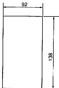
パネルカット寸法
