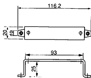
取付金具寸法
